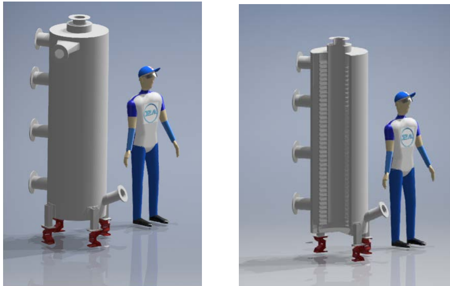
Kuva 3. Hitaan pyrolyysin prosessilaite, tekninen toteutus ja mittakaava.
